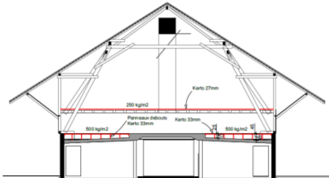
Coupe transversale
